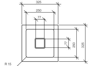
WT.Q1 325 Wall Basin 4.5 ltr capacity 9500778
