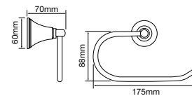
D Toilet Roll Holder
